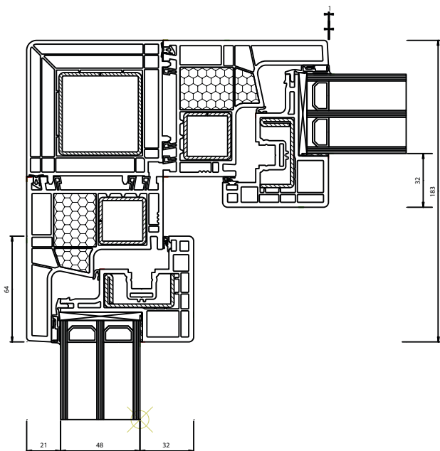
Cuplaj 90 gr.
