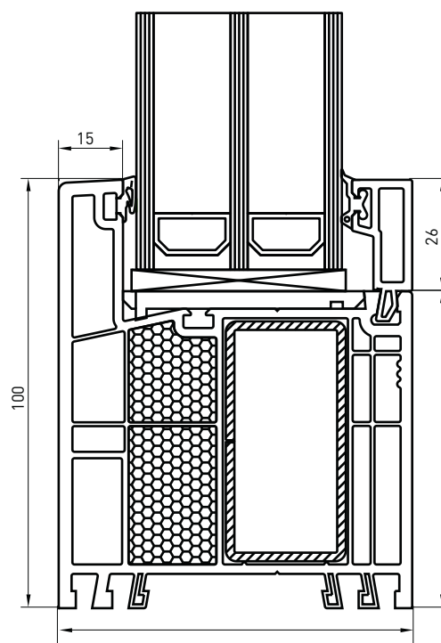
Canat fix
