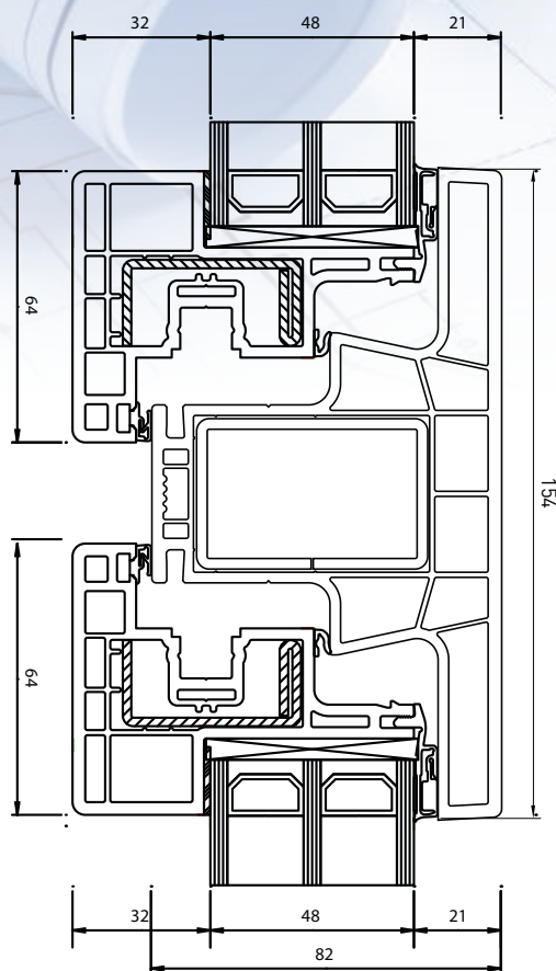
Modul 2 canate mobile cu montant fix
