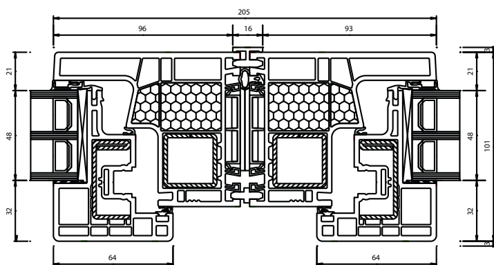
Cuplaj H
